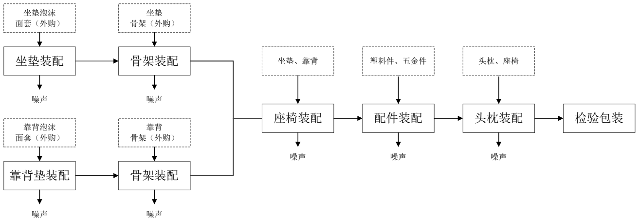
图 3-2 营运期工艺流程及产污情况图
