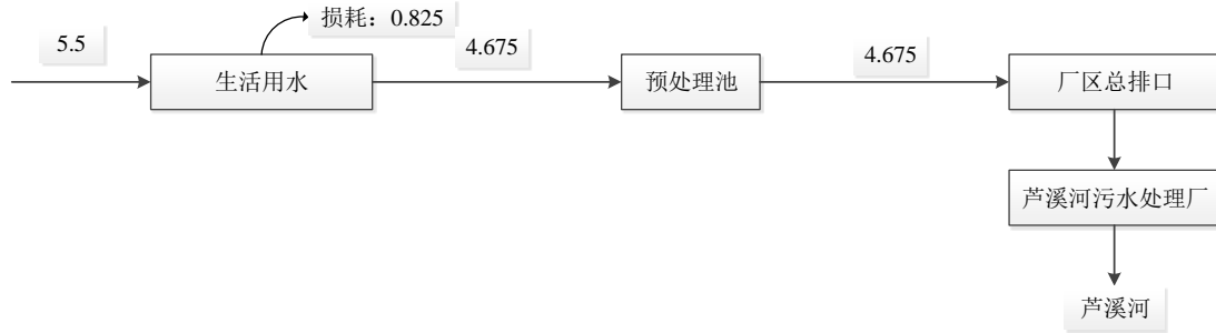
图 3-1 水量平衡图（单位：m 3 /d）
